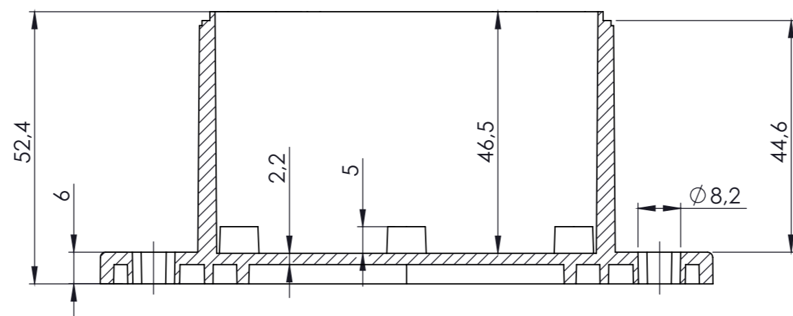
PRZEKRÓJ A-A
