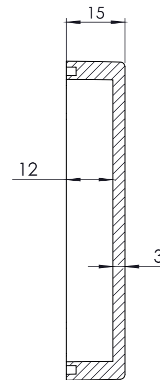
PRZEKRÓJ A-A
