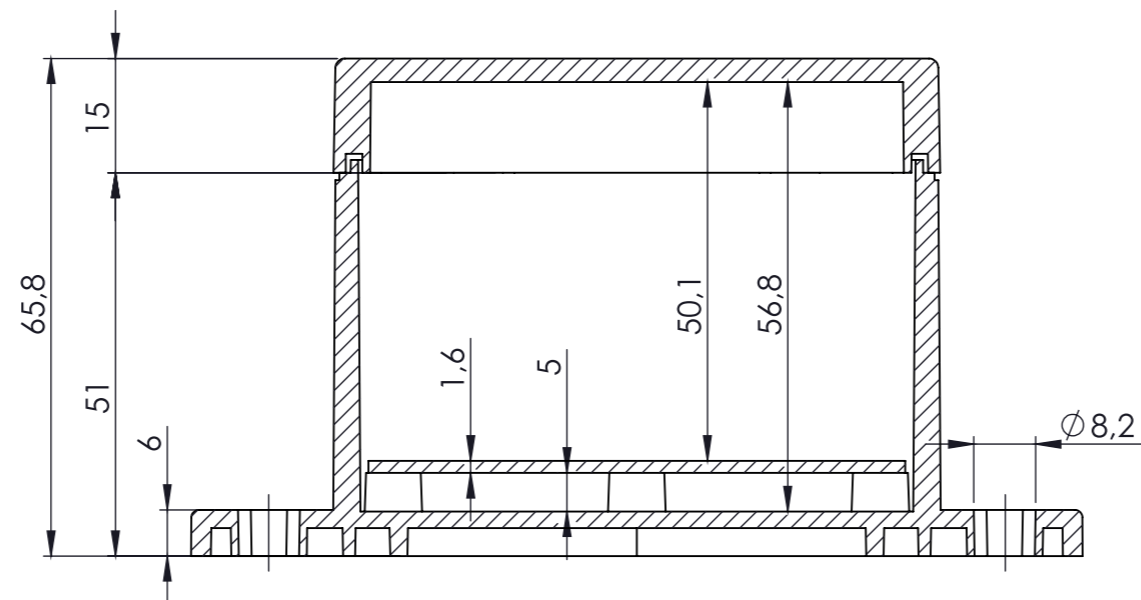
PRZEKRÓJ A-A
