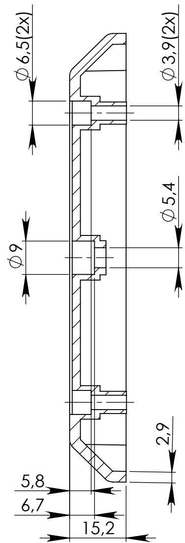
PRZEKRÓJ A-A
