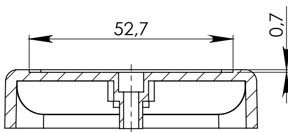
PRZEKRÓJ B-B
