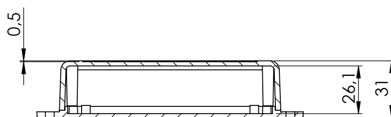
PRZEKRÓJ A-A
