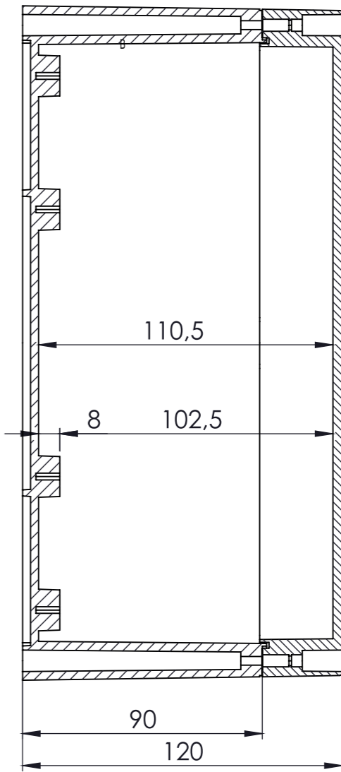
PRZEKRÓJ A-A
