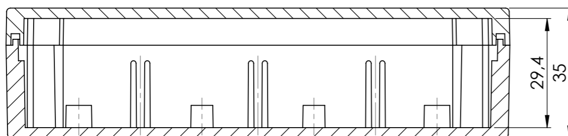
PRZEKRÓJ A-A
