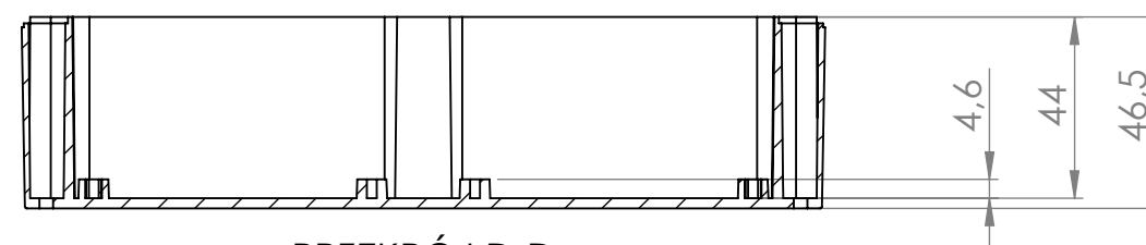
PRZEKRÓJ D-D
