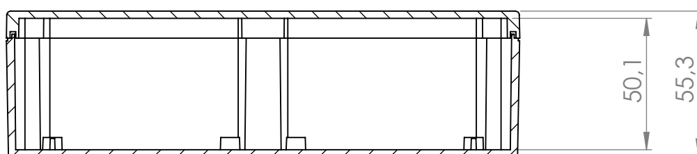
PRZEKRÓJ A-A
