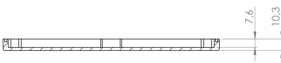
PRZEKRÓJ E-E
