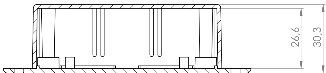
PRZEKRÓJ D-D
