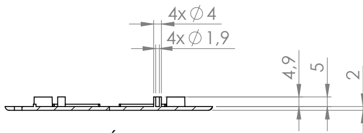
PRZEKRÓJ C-C
