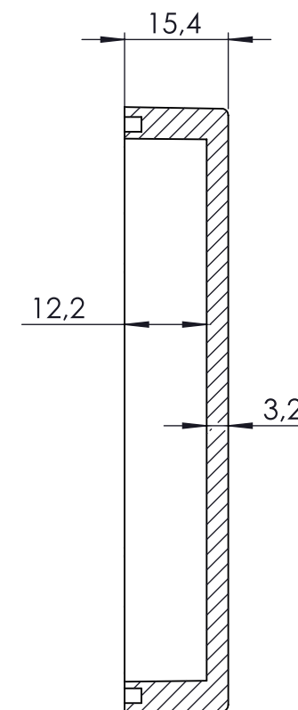
PRZEKRÓJ A-A
