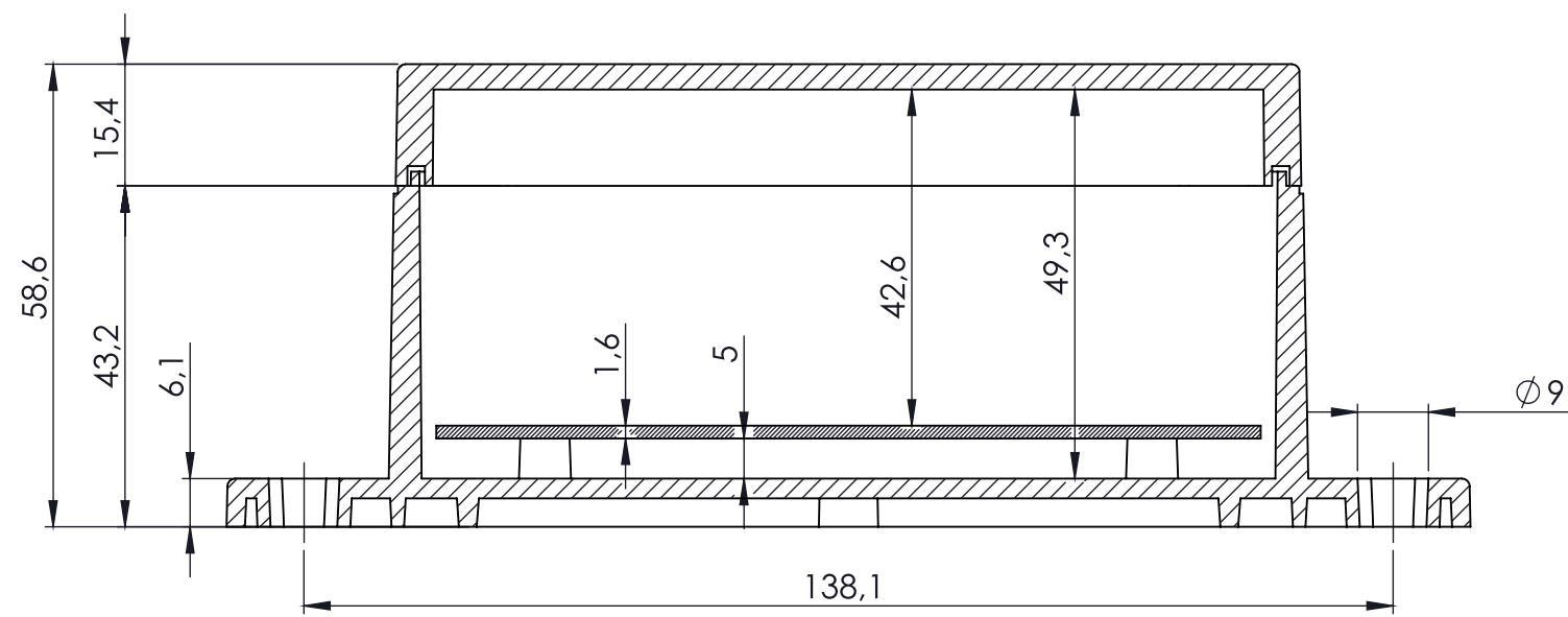
PRZEKRÓJ A-A
