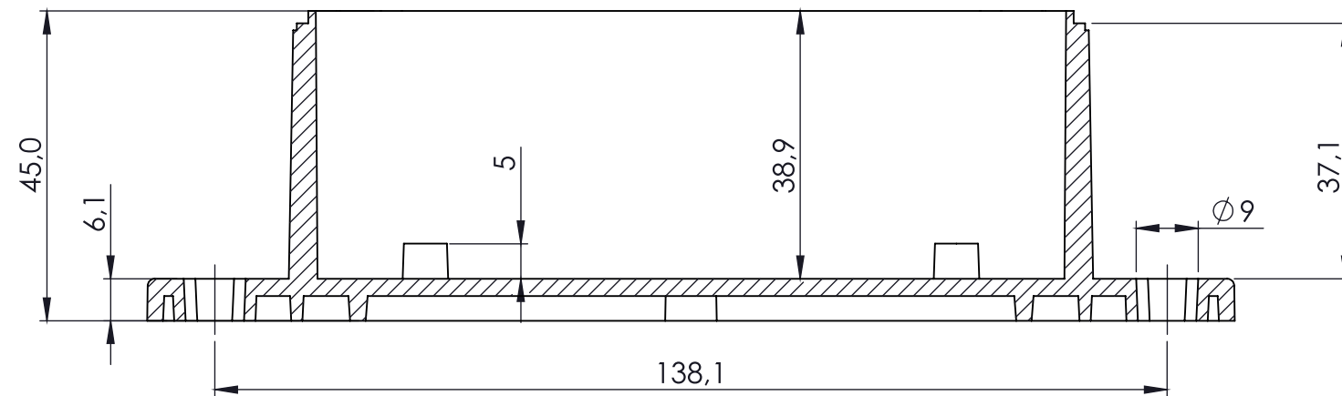
PRZEKRÓJ A-A
