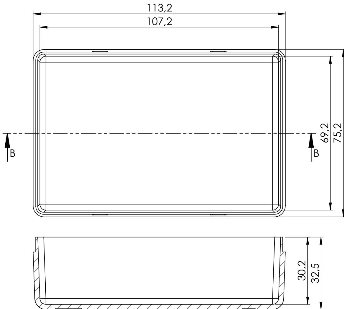
PRZEKRÓJ B-B
