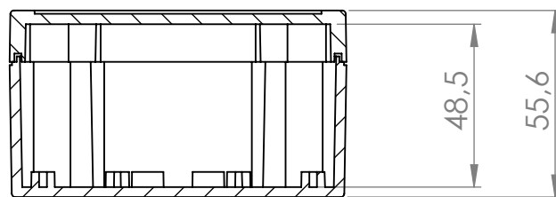
PRZEKRÓJ A-A
