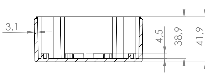
PRZEKRÓJ B-B
