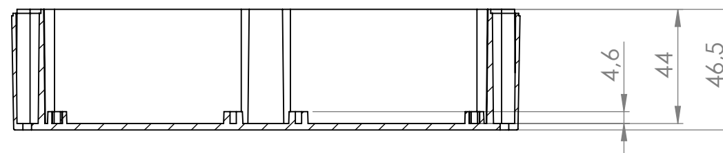
SECTION D-D
