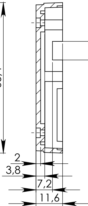
PRZEKRÓJ B-B
