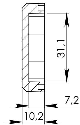
PRZEKRÓJ B-B
