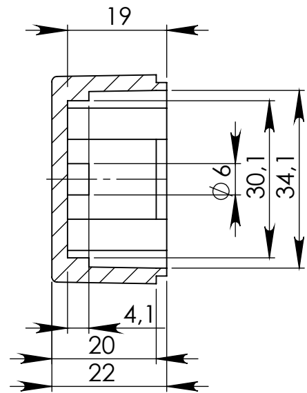
PRZEKRÓJ A-A
