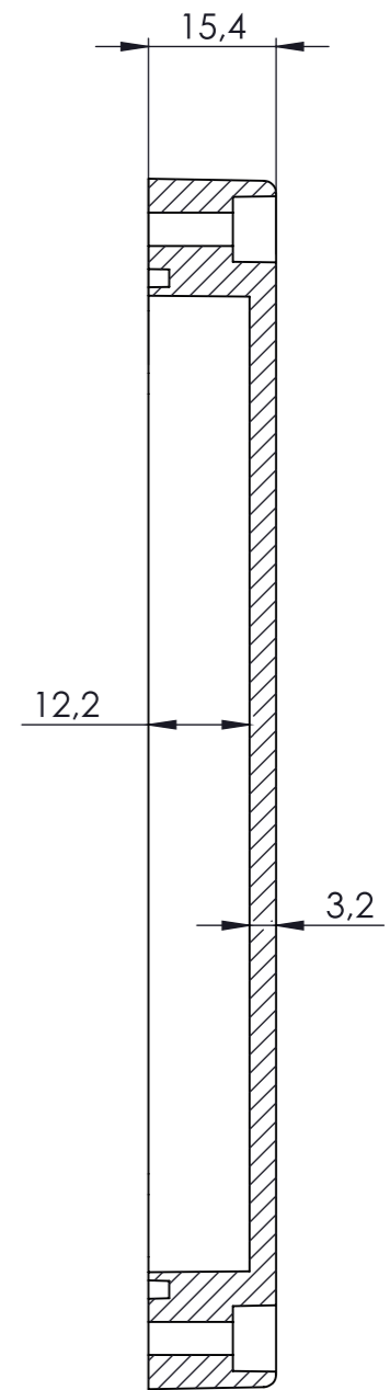
PRZEKRÓJ A-A
