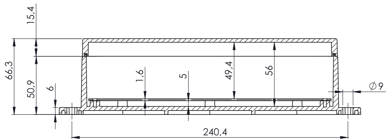
PRZEKRÓJ A-A
